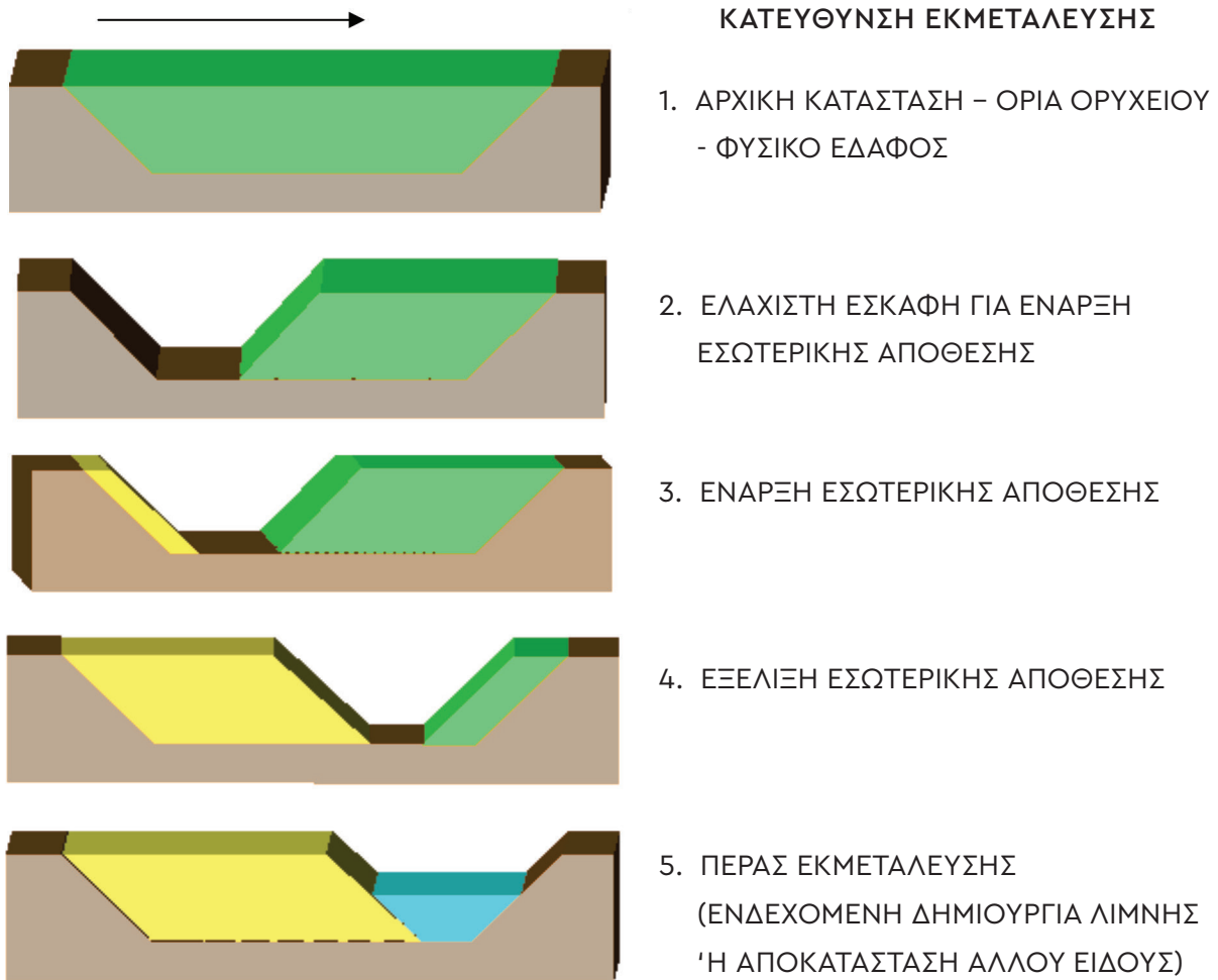
Σχήμα 3. Στάδια εξέλιξης της εκμετάλλευσης ορυχείου
